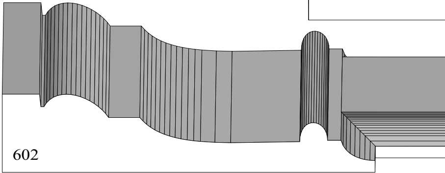
BA 602 3/16" x 3-15/16" BA 602B Cope BA 602C Mullion
